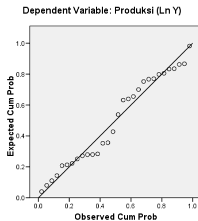
Gambar 1. Grafik Scatter Plot Uji Normalitas
