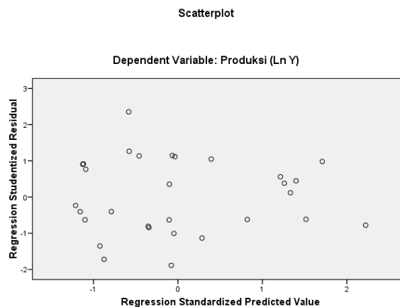
Gambar 2. Grafik Uji Heteroskedastisitas Sumber : Data Primer, 2017 (Diolah)
